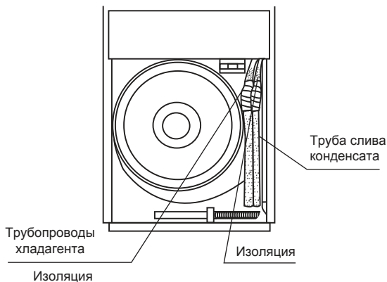
Отверстие для трубопроводов на боковой стороне внутреннего блока
